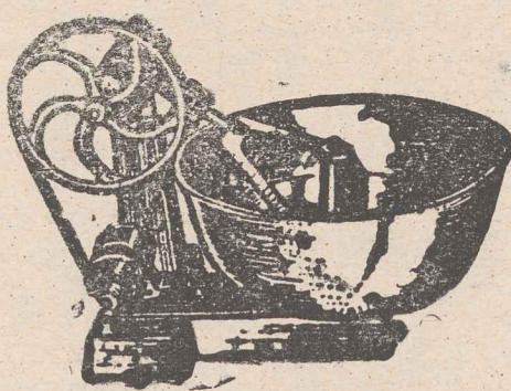
ΚΥΛΙΝΔΡΟΣ ΕΥΡΩΠΑΪΚΟΥ ΤΥΠΟΥ ΑΥΤΟΜΑΤΟΣ ΑΝΕΥ ΕΡΓΑΤΟΥ, ΜΕ ΑΥΞΟΜΕΙΩΣΙ ΤΗΣ ΑΠΟΣΤΑΣΕΩΣ ΤΩΝ ΔΥΟ ΚΥΛΙΝΔΡΩΝ.
