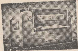
ΚΥΛΙΝΔΡΟΣ ΕΥΡΩΠΑΪΚΟΥ ΤΥΠΟΥ ΑΥΤΟΜΑΤΟΣ ΑΝΕΥ ΕΡΓΑΤΟΥ, ΜΕ ΑΥΞΟΜΕΙΩΣΙ ΤΗΣ ΑΠΟΣΤΑΣΕΩΣ ΤΩΝ ΔΥΟ ΚΥΛΙΝΔΡΩΝ.
