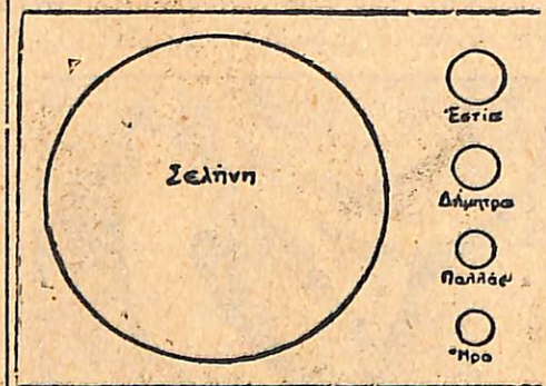
Σχετικὰ μεγέθη (ἀνάλογος τῆς διαμέτρου αὐτῶν) τῆς σελήνης καὶ τῶν τεσσάρων μεγάλων ἀστεροειδῶν
