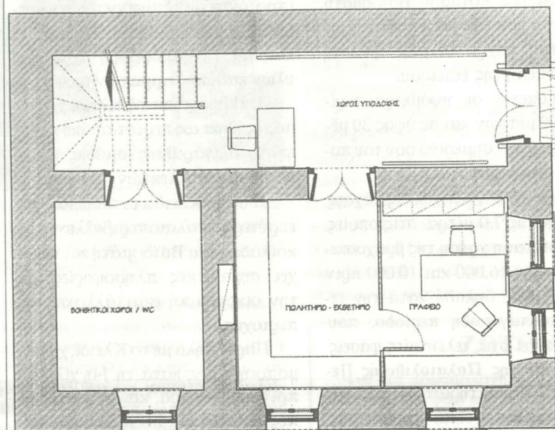
ΚΑΤΩΦΗ ΙΣΟΓΕΙΟΥ - ΚΛ. 1:50
