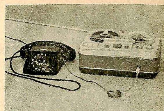
Είς όν 1. Έγγραφή Τηλεφωνικής κλήσεως με την βοήθειαν συσκευής Μαγνητοφώνου Τελεφούνκεν KL 65 X και τηλεφωνικού πηνίου
