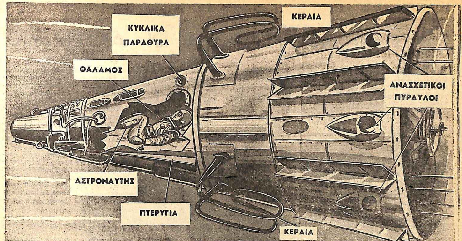
Τὸ σχέδιο αὐτὸ πὸ δημοσιεύθηκε σὲ ρωσικὴ ἐφημερίδα, δίνει μιὰ ἰδέα τοῦ διαστημοπλοίου «Βοστόκ». Ἡ βάση τοῦ κῶνου εἶναι ὁ τελευταῖος «δρόμος» τοῦ προωθητικοῦ πυραύλου καὶ περιέχει τὶς πολὺπλοκες συσκευὲς τηλεπικοινωνίας καὶ κλιματισμοῦ τοῦ θαλαμίσκου. Στὴν κορυφὴ τοῦ κῶνου περιέχεται ὁ θαλαμίσκος τοῦ κοσμοναῦτη πὸ, ξαπλωμένος ἀνάσκελα, μπορεῖ νὰ βλέπει τὸν ἔξω κόσμὸ ἀπὸ μιὰ ζώνη κυκλικῶν παραθύρων.
