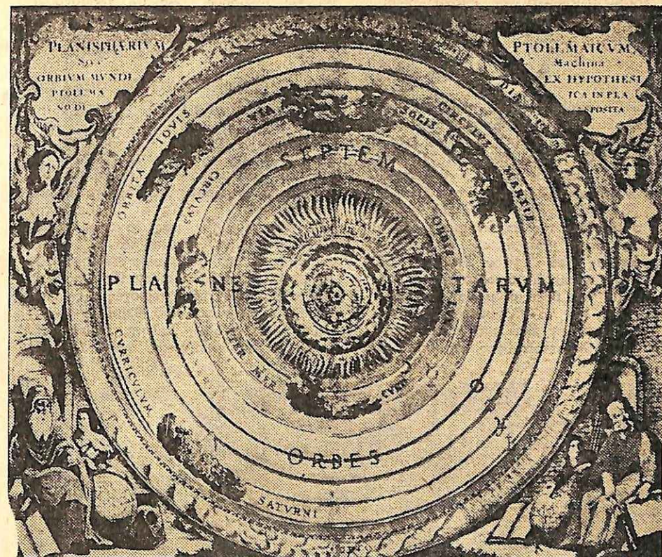
Το Σύμπαν, όπως το φαντάστηκε ο Πτολεμαίος. 'Ανασκευάζοντας αυτή την αρχαία κοσμολογική αντίληψη, ο Κοπέρνικος κι' ο Γαλιλαίος έθεσαν τις βάσεις των νέων επιστημονικών αντιλήψεων, που αποκαρυσώνονται με τις τομηρές θεωρίες ενός Νταβίντφ ή ενός Τζίλδαρυ.
