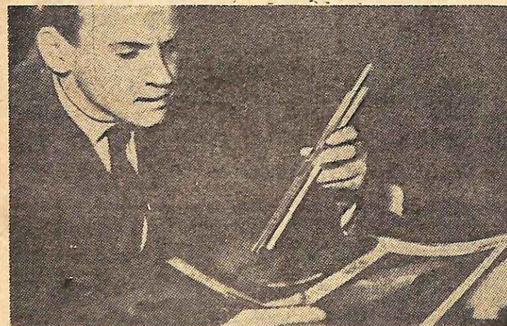
Ο Βίκτωρ Νταβίντωφ, ο νεαρός Σοβιετικός αστρονόμος που μελετά τα προβλήματα του "Αρη κάτω από το φως της θεωρίας ότι το νερό είναι ιδρώτας των πλανητών.
