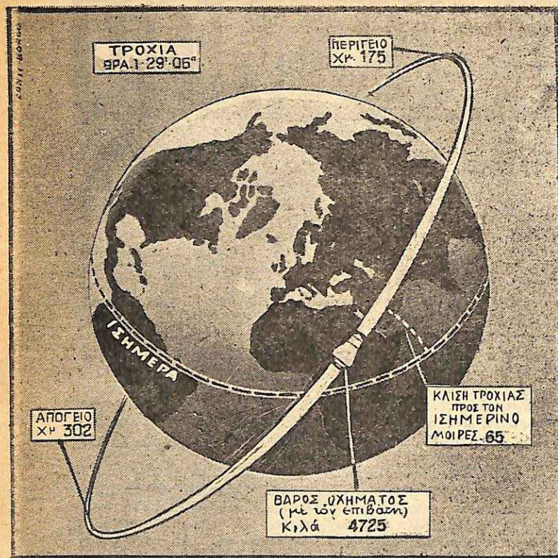
Η τροχιά του ρωσικού διαστημοπλοίου «Βοστόκ» γύρω από τη Γη.
