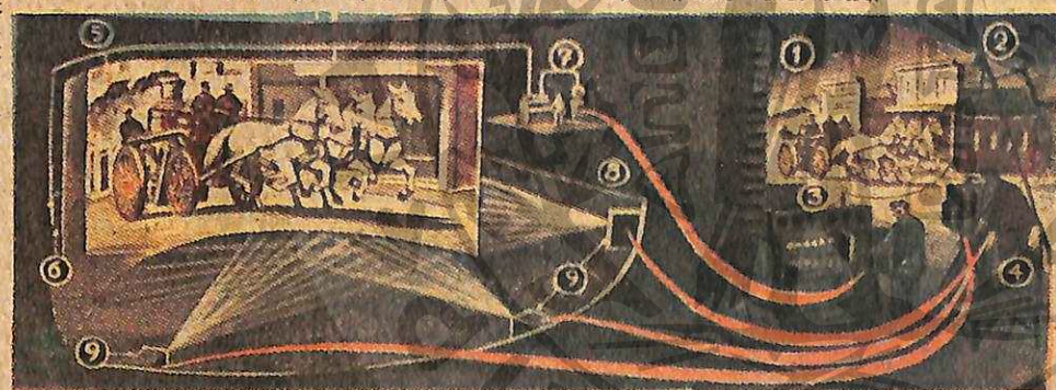
Σχηματικό διάγραμμα του γυρίσματος καί της προβολής ενός φιλμ με τη νέα μέθοδο. 1) Στούντιο. 2) Μικρόφωνο. 3) Μηχανήμα φωνολήψις. 4) Τριπλή κινηματογραφική μηχανή. 5) Όθονη προβολής. 6) Πέντε μεγάφωνα. 7) Άπόδοσις ήχου. 8) Φιλμ του ήχου. 9) Μηχανές προβολής.
