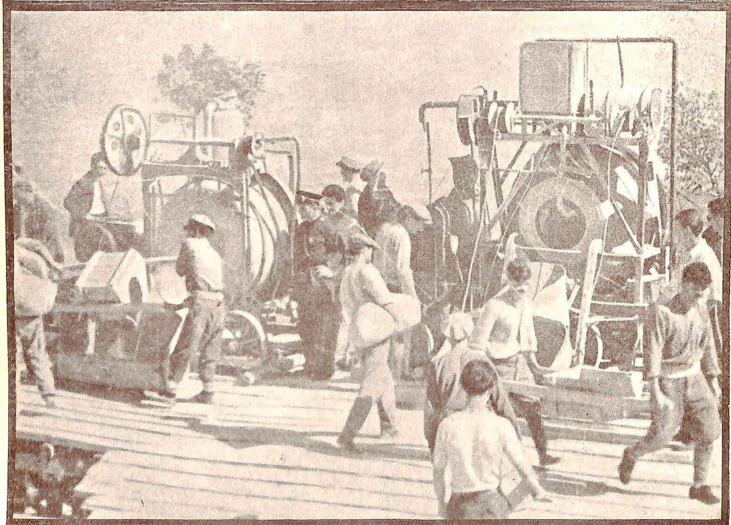
Από τα οχυρωματικά έργα της Ελληνικής γραμμής Μιζινώ «Ι. Μεταξάς». Ανω: Στόμιον πολυβολείου. Κάτω: Κατασκευή εξωτερικών έργων.
