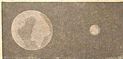
Συγκριτικό μέγεθος Γης και Σελήνης
