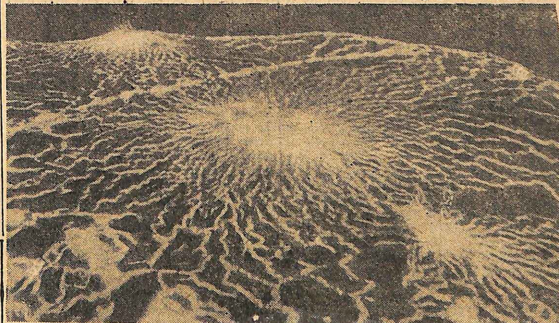
Ἠφαίστειον θεώμενον ἀπὸ ἀεροπλάνου, κατόπιν ἐκρήξεως. Διακρίνονται ἀκέρμη τὰ ρυάκια τῆς λάβας.
