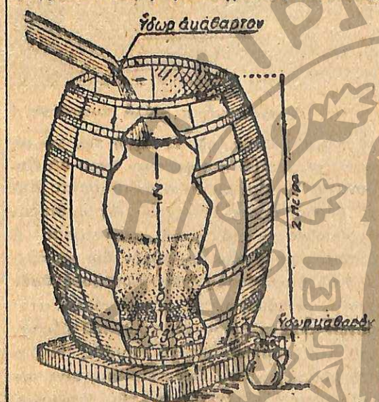
Βαρέλιον — διῦλιστήριον κατάλληλον δι' ἐξοχὰς. — α, σειρά τοῦδλων. β, σειρά λίθων. γ, χάλικες. δ, ὡμίς χονδρῇ. ε, ἄμμος λεπτῇ. ζ, χώρος διὰ τὸ ὕδωρ.
