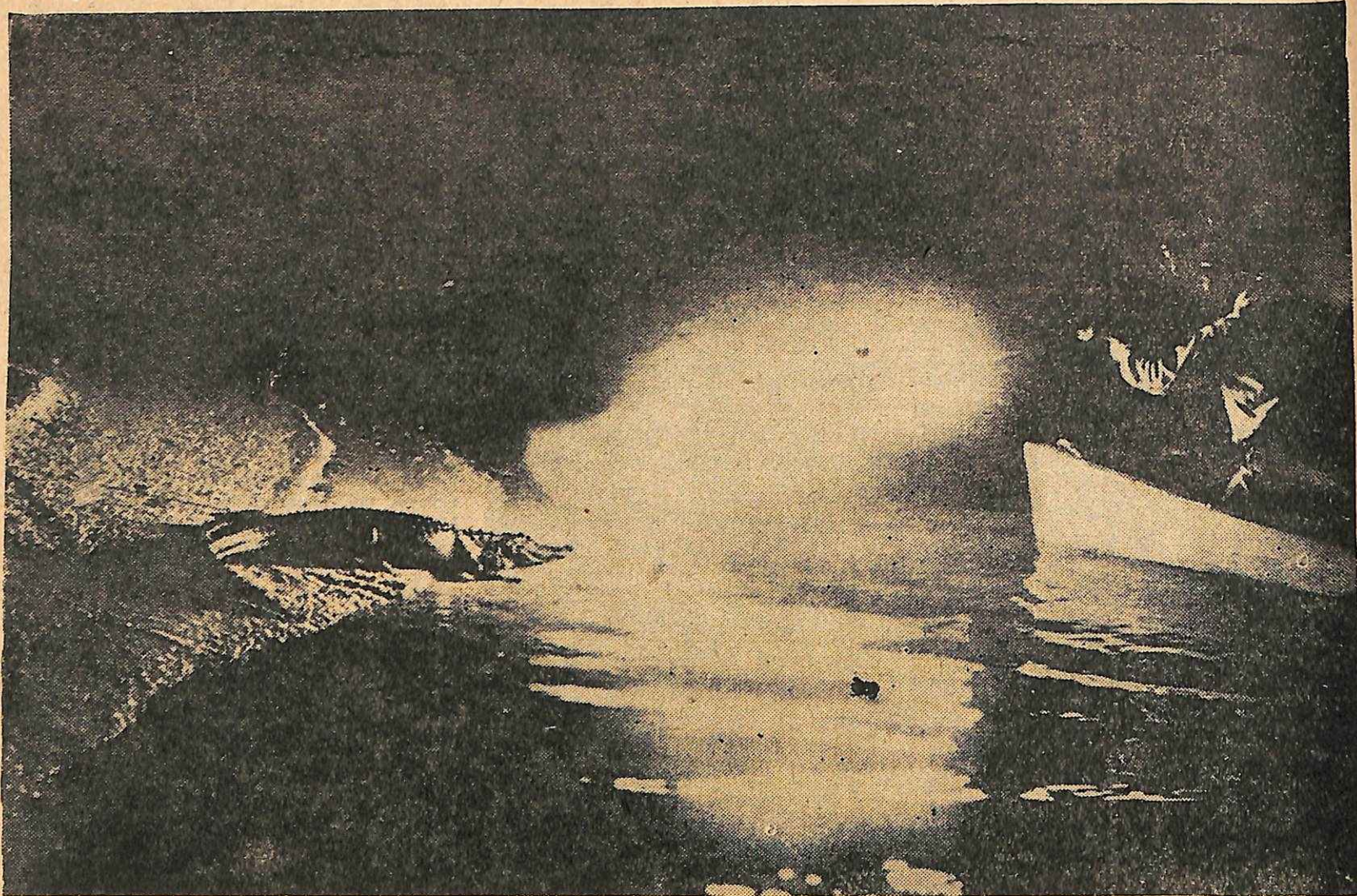
Τὸ μαγνήσιον φωτίζει τὸ σκοτάδι καὶ ξαφνιάζει τοὺς κροκοδείλους
