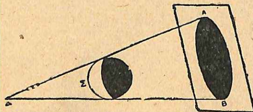
(Φ=φωτεινὴ ἀκτίς. Σ=παρεντιθέμενον σῶμα. AB=συνὴ τοῦ σώματος Σ.)
