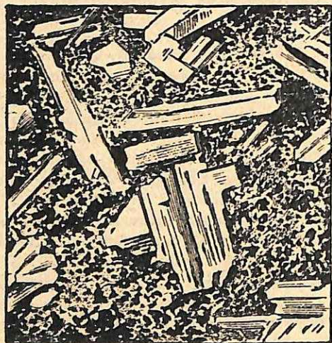
1.—Στρώματα γρανίτου.
