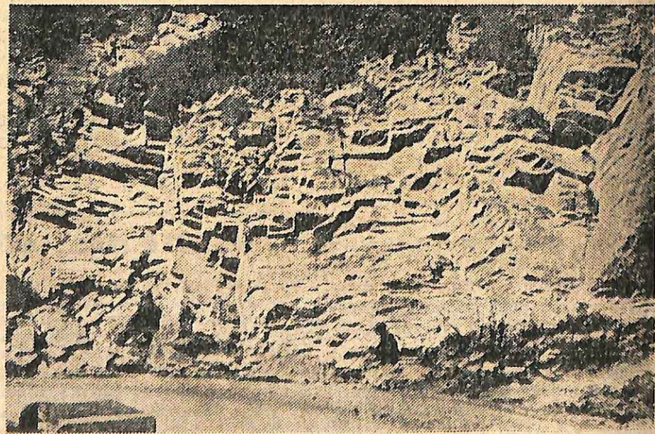
3.—Συντρίμματα ἀρχαίων ἀσβεστολιθικῶν στρωμάτων εἰς τὸ Τεφουναίστεν τῆς Ἑλβετίας.
