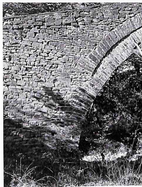
((Φωτ. 28-2) Λεπτομέρεια αριστερού ακροβάθρου «γέφυρας Πεκλαρίου Μπούσης», όψη ανάντης, όπως ήταν το 2016. Διακρίνεται το λευκό βοηθητικό στεφάνι του τόξου και η γραμμή διαχωρισμού στην τοικοδομία του στηθαίου. [Λήψη: Θωμά Β. Ζιώγα, 09-08-2016].
