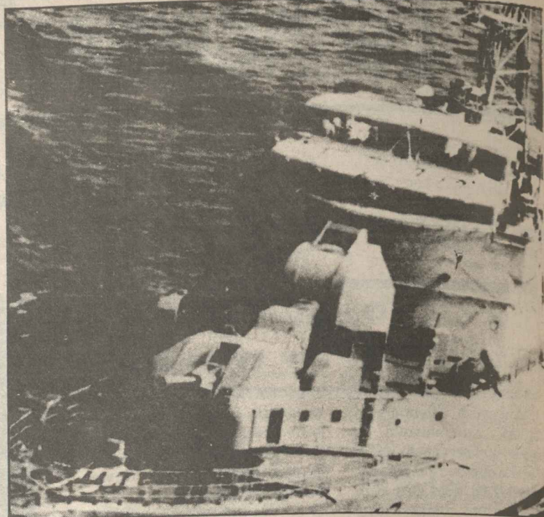
Η γαλλική φρεγάτα «Τρότε», ενώ πλέει στον Περσικό Κόλπο
