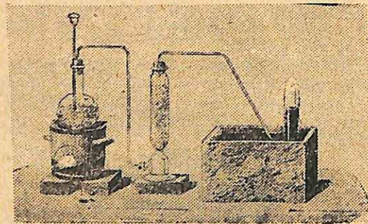
Συσκευή παραγωγῆς ξηρᾶς ἀμμωνίας
