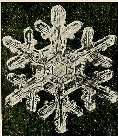
Σχεδιάσμα χιονοκρυστάλλου
