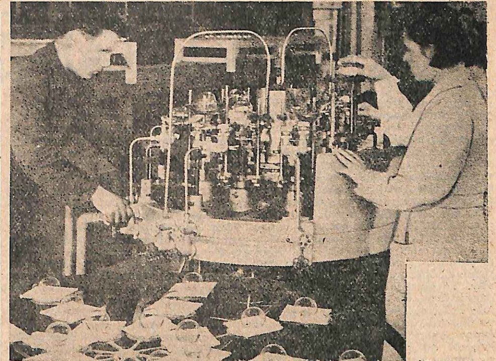
Μὲ τὸ μηχανήμα αὐτὸ τοποθετεῖται τὸ ὑάλινον ποδάρι τοῦ λαμπτήρος μέσα στὴν ὑαλινὴν σφαῖραν. Ἐμπρὸς διακρίνονται οἱ λαμπτήρες ἐκείνοι εἰς τοὺς ὁποίους εἰσῆχθη τὸ ποδάρι.
