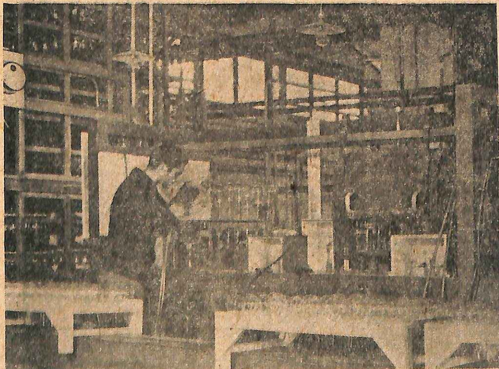
Ἀφοῦ τὸ ποδάρι εἰσῆχθη εἰς τὴν ὑαλινὴν σφαῖραν καὶ ὁ λαμπτήρ ἔλαβε ἤδη τὴν πρῶτην του μορφήν, μὲ τὸ εἰκονιζόμενον ἐργαλεῖον ὁ ἐργάτης ἀφαιρεῖ τὸν ἀέρα τοῦ λαμπτήρος καὶ κατόπιν τὸν γεμίζει μὲ ἀδρανὲς ἀέριον.
