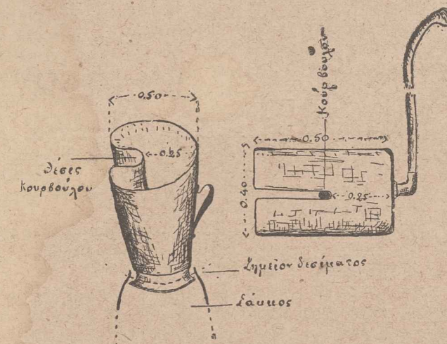
Χωνί και φτυάρι χρησιμοποιούμενα διά την συλλογήν του σκαθαριου της άμπέλου.
