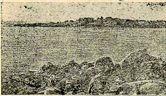
Πλημμυρίδα: 'Η θάλασσα έχει κατακλύσει την ξηρά και έχει σχηματίσει νησάκια.
