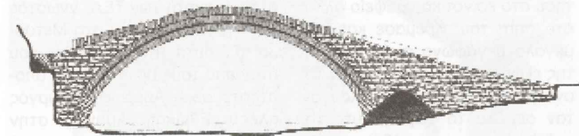
(Φωτ. 18-2) Η «γέφυρα Κλειδωνιάς» σε αποτύπωση και σχέδιο του 1987. Κατάντη όψη. [Πηγή: «Τα πετρογιόφυρα της Ηπείρου», Ιωάννινα 2012/3, σελ. 76, έκδοση ΥΝΜΤΕΗ (Περιφέρεια Ηπείρου)].
