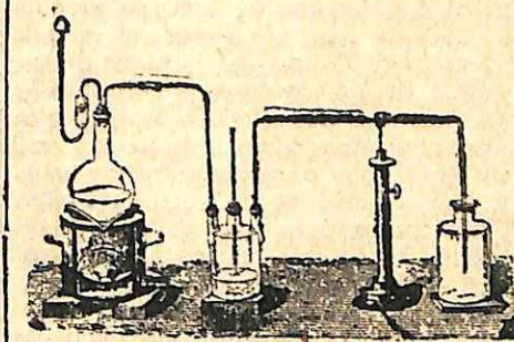
Συσκευή διὰ τὴν παρασκευὴν τοῦ χλῶριου.
