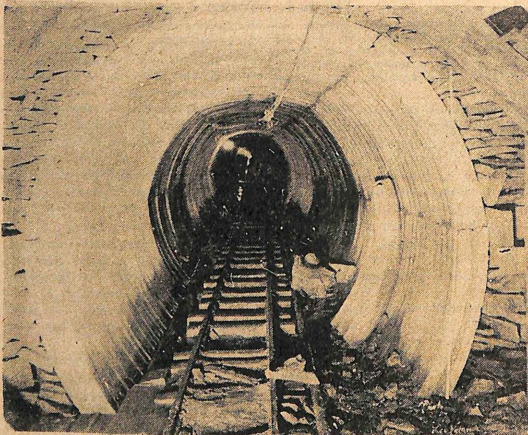
Τμήμα τῆς μεγάλης σήραγγος (ὕψος 2.48 μ. καὶ πλάτος 2.30) ἐπενδεδυμένης κατὰ πυκνά διαστήματα διὰ δακτυλίων ἐκ σκυροκονιάματος. Ἡ φωτογραφία ἐλήφθη ὑπὸ ἀκόμῃ κατεσκευάζετο ἡ σήραγξ.
