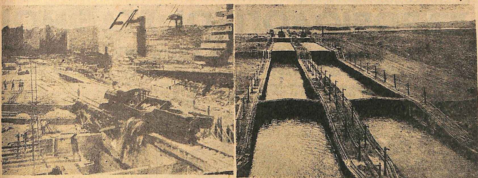
Ἡ μεταξὺ τῆς λίμνης Γκατοῦν καὶ τοῦ Ἀτλαντικοῦ περιοχή καὶ τὰ τὸ διάστημα τῶν ἐργασιῶν καὶ ὡς ἔχει τώρα μὲ τὰς τρεῖς κλεισίαντες συνολικοῦ μήκους δύο καὶ ἡμίσεος χιλιομέτρων.
