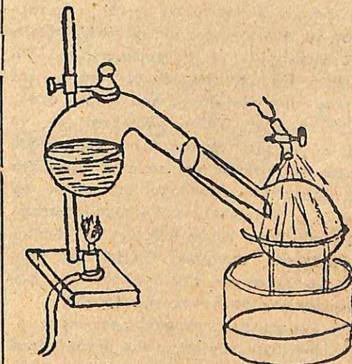
Συσκευή παρασκευῆς νιτρικοῦ ὀξέος εἰς τὰ χημικὰ ἐργαστήρια.
