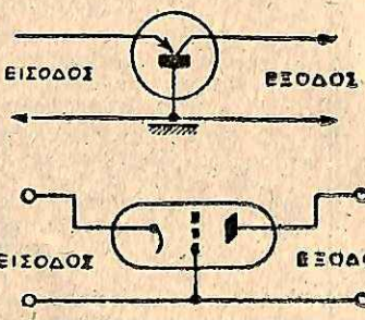
Σύγκρισις ενισχυτού γερμανίου (άνω) και λυχνίας (κάτω)
