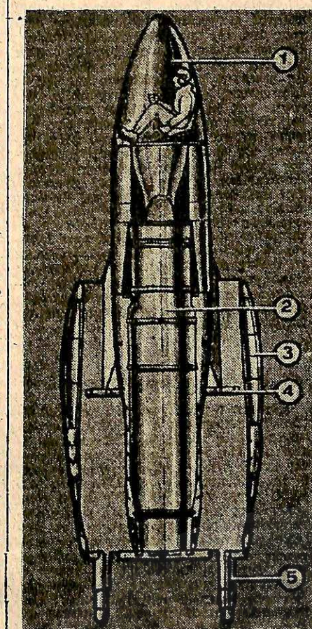
Κολεόπτερον, ή νέα πτητική συσκευή με τὰ κυκλϊκά πτερά. 1 θάλαμος πιλότου, 2 πυ- ραύλος, 3 κυκλϊκα πτέρυγες, 4 διάφραγ- ματα, 5 στηρίγματα
