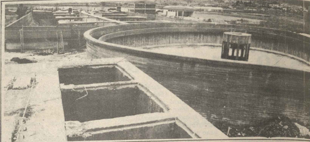
Μία από τις δεξαμενές προτοβάθμιας καθίζησης
