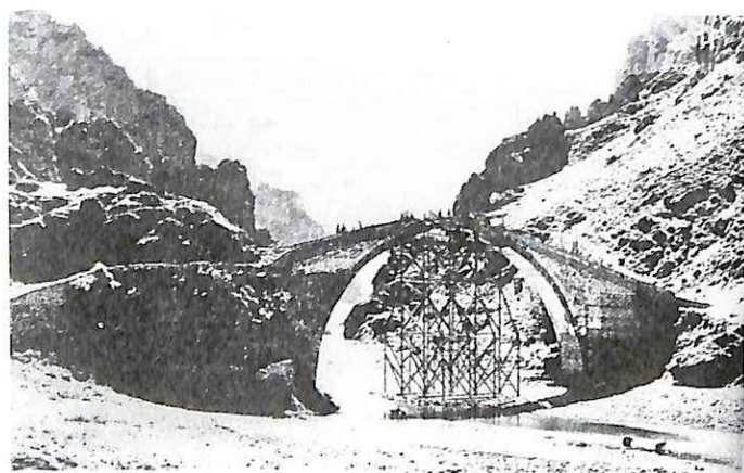
(Φωτ. 19-2) Κατάντης όψη της «γέφυρας Κόνιτσας» το 1913. Επισκευή βλάβης κορυφής, από τον κανονιοβολισμό εκ μέρους των Τούρκων. Δεν διακρίνεται το αυλάκι του μύλου στη δεξιά όχθη (προς Κόνιτσα). [Πηγή: Φωτογραφικό Αρχείο Freed Boissonas, 1913].
