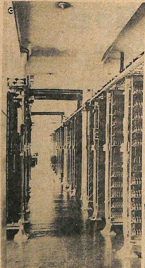
Διάδρομος εις την αίθουσαν επιλογών του Κεντρικού Τηλεφωνικού Κέντρου 'Αθηνών.
