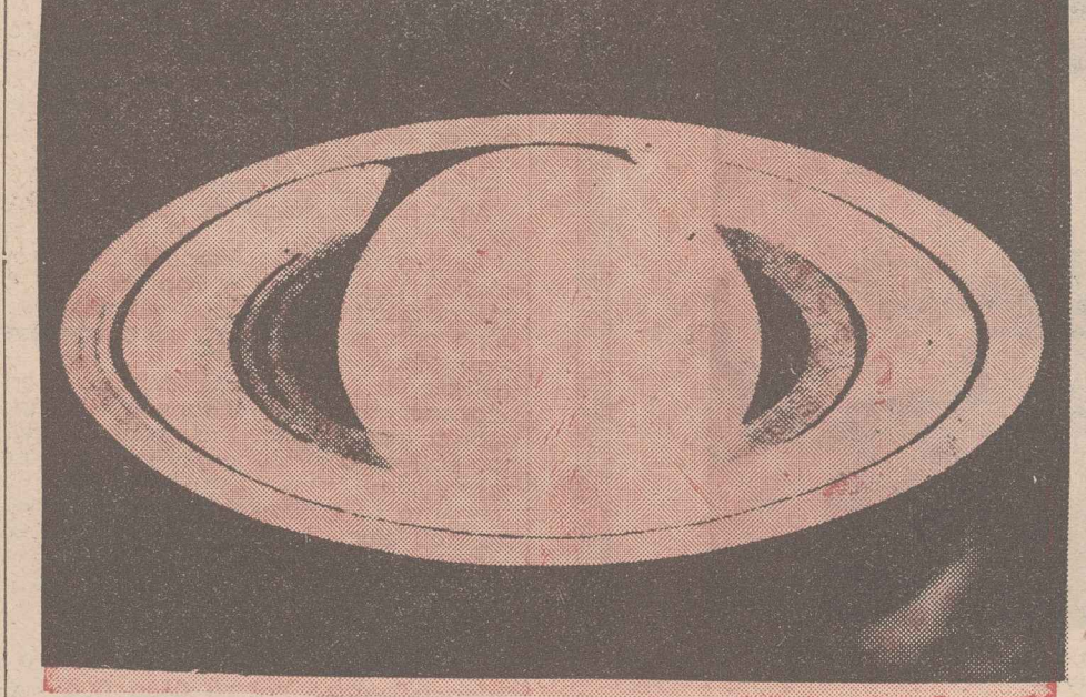
Φωτογραφία του πλανήτη Κρόνου μετά των τριών δακτυλίων του. Κατά το 1937 θ' άρχίσουν βαθμιαίως να διακρίνονται οι τρεις δακτύλιοι, διότι το 1936 τα έπίπεδα των εφρίκονται εις το αυτό έπίπεδο με την όπτική άκτίνα και δεν έχωρίζοντο.
