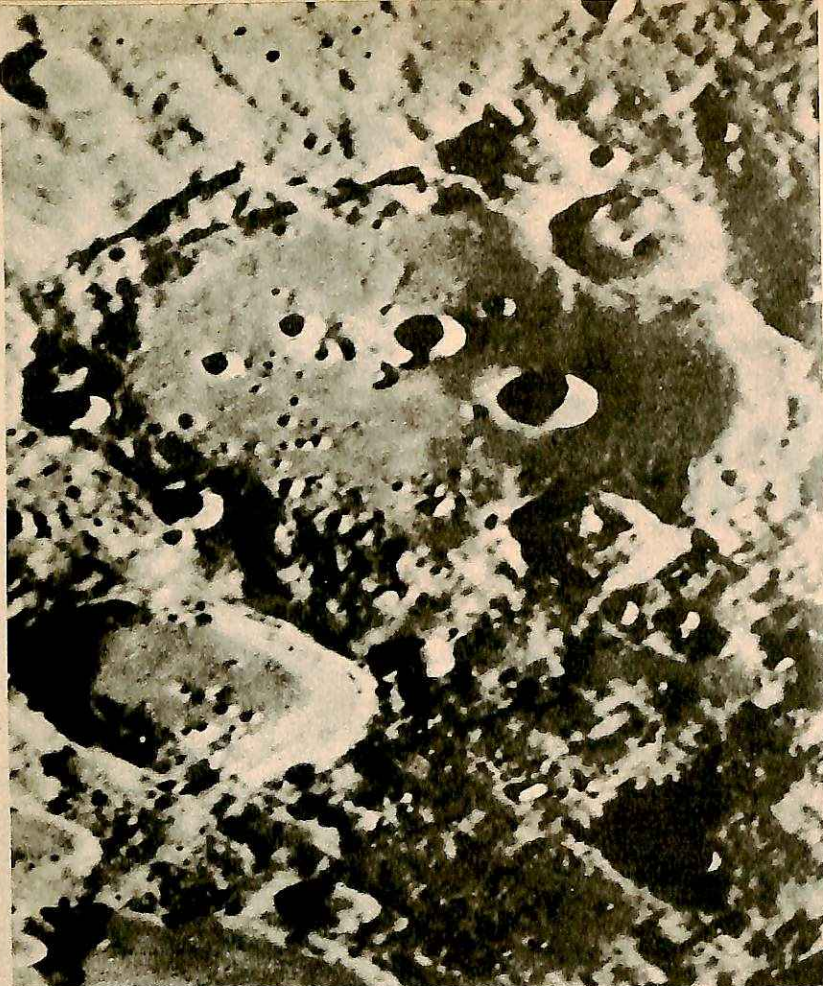
ΜΙΑ ΕΞΑΙΡΕΤΙΚΑ καθαρή φωτογραφία του νοτίου πόλου της Σελήνης, όπως την έδωσε το 'Αστεροσκοπείο των Παρισίων. 'Ο πύραυλος για να φθάσει στον δορυφόρο μιας θα πρέπει να διανύσει την φανταστική απόσταση των 384.000 χιλ. 'Η πραγματοποίηση του όθλου εκτός από τις άλλες άπρσιμέτρητες συνέπειες, θα βοηθήσει τους αστρονόμους να λύσουν δυο αινίγματα που τους απασχολούν από παλιά. Τι είναι πραγματικά το Μέγα Τείχος μήκους 15 χιλ. που διακρίνεται σ' ολόκληρη την επιφάνεια της Σελήνης και τι είναι αυτός ο μυστηριώδης Κρατήρ του Κοπερνίκου;
