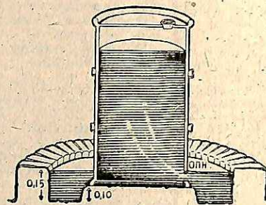
Ποτίστρα με σιδερένιο βαρέλι (τομή).
