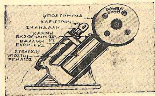
Σχηματικὴ παράστασις τοῦ τρόπου λειτουργίας τοῦ ἐιδικοῦ πυροβόλου διὰ τὴν ἐκσφενδόνισιν τοῦ βομβῶν βυθοῦ.
