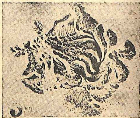
Ακανόνιστη ήλιακή κηλίς. (Αι διαστάσεις αὐτῆς έν συγκρίσει με την Γην).
