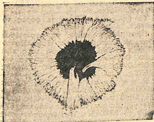
Κανονική ήλιακή κηλίς. (Διακρίνεται ή σκιά και τό περισκίασμα).
