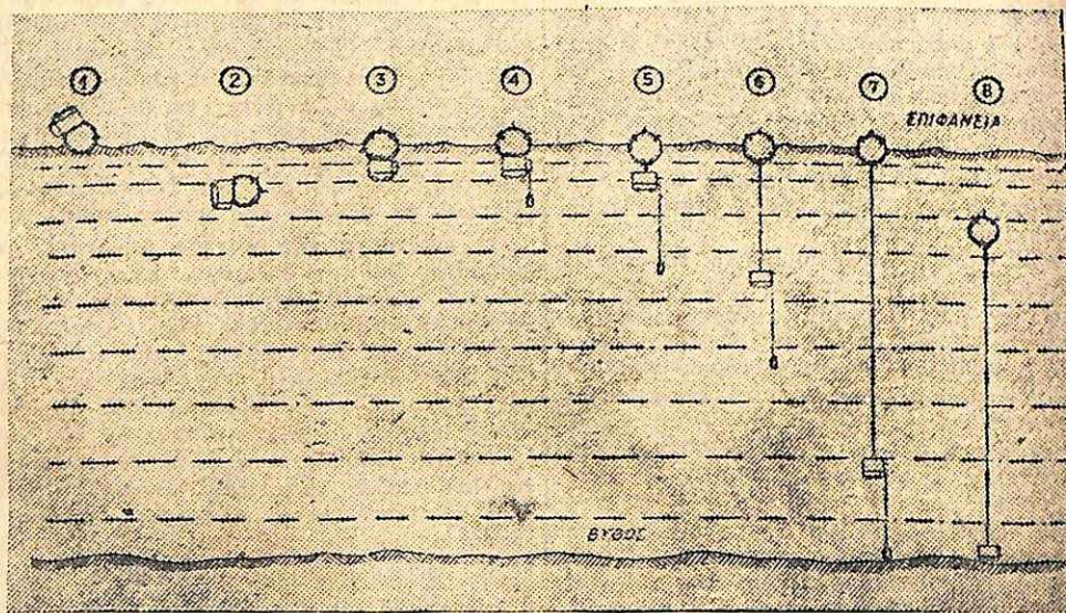
Διάγραμμα δεικνὺν τὰ διαδοχικὰ στάδια ποντίσεως νάρκης
