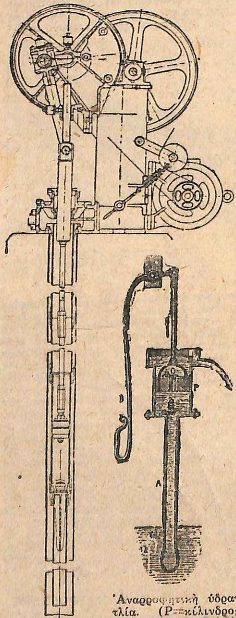
Ἀναρροφητικὴ ὑδραντλία. (P=κύλινδρος, A=σωλήν, β=βαλβίς, B=μολύβδος λειτουργίας φρεάτων).
