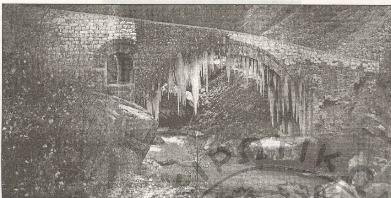
Η γέφυρα «ΦΙΛΟΥ» επί του «ΧΡΟΥΣΙΑ», παραποτάμου του Αράχθου με κρεμασμένους πάγους στο θόλο της στις 6 Ιανουαρίου 2002
