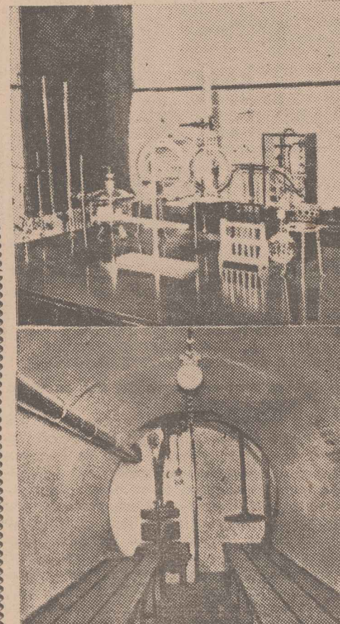
Άνα : Τό εργαστήριον διά τών ά- μοφοβερικών έλεγχόν το καταφυγί- ου και της άναενοώσεως του άέρος. Κάτω : Μία στοά του άντιαεροπο- ρικού καταφυγίου.
