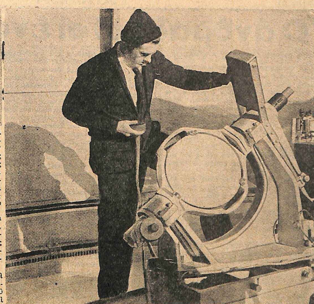
Τὸ κατόπτρον τοῦ ἡλιακοῦ ἀστεροσκοπεῖου τοῦ Μάουντ Οὐίλσον, τῇ βοηθείᾳ τοῦ ὁποῖου λαμβάνονται αἱ φωτογραφίαι τοῦ ἡλίου.
