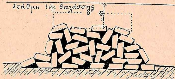
Σχέδ. III. — Μῶλος Λευκάδος Τομή. — Κλίμαξ 1/200
