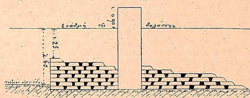
Σχ. I. — Κρηπιδώμα Ρηνείας Κλίμαξ 1/100
