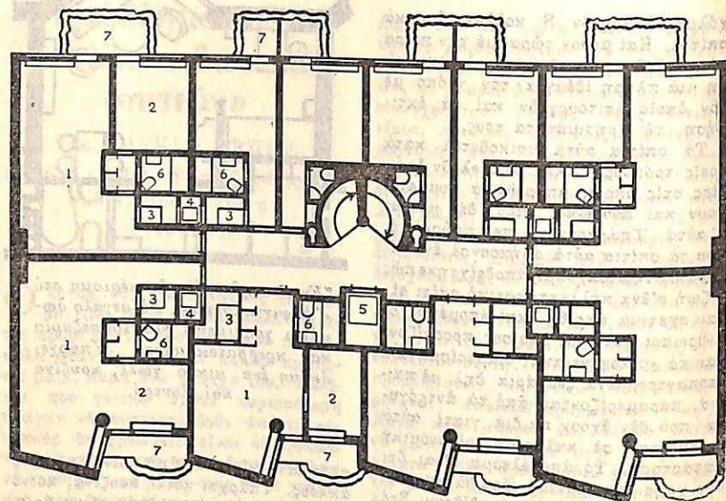
Κάτοψη του πρώτου κολλεκτιβιστικού σπιτιού της Στοκχόλμης, έργο του αρχιτέκτονος Σβέν Μαρκέλιους: 1) Καθημερινό δωμάτιο. 2) Κρεβατοκάμαρα. 3) Κουζίνα. 4) Άσανσέρ για τα φαγητά. 5) Άσανσέρ. 6) Λουτρό. 7) Βεράντα.
