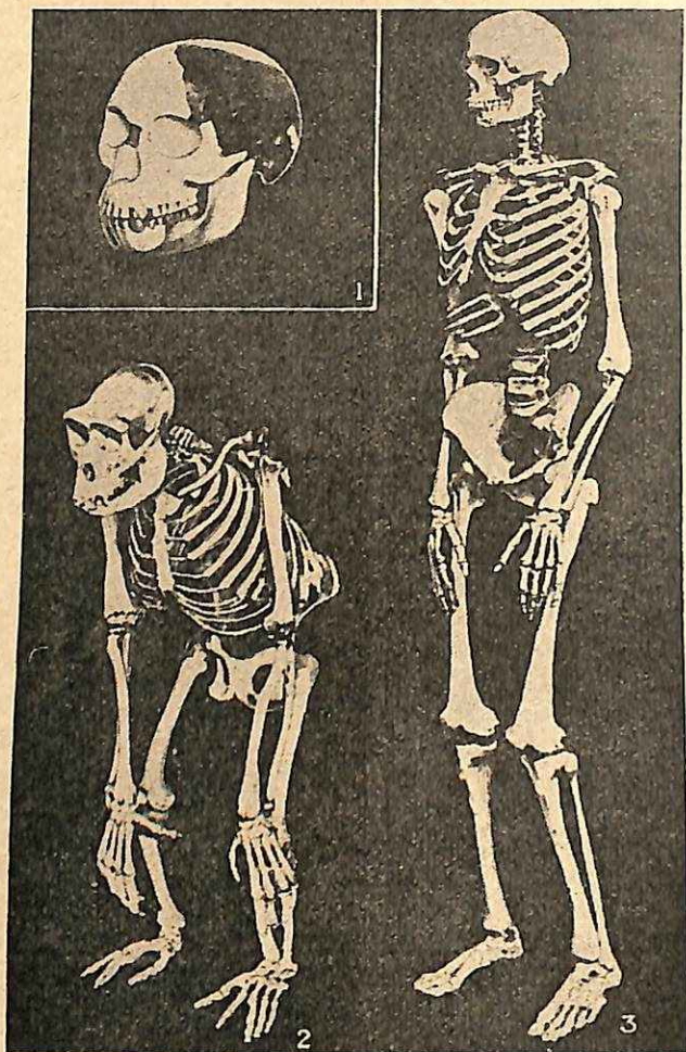
Σκελετὸς ἀνθρώπου (3) ἐν συγκρίσει πρὸς σκελετὸν χιμπατζῆ (2). Τὸ εὐρεθὲν ἐν Πιλντνόουν τοῦ Σάσσεξ κρανίον (1) συναρμωσθὲν, ἀποδιδόμενον δὲ εἰς τὸν Ἡωάνθρωπον.
