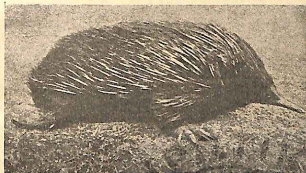
Ἄλλο ἐπιβιώσαν ζῷον τοῦ ἐξαφανισθέντος τύπου· φωτοζον μαστοφόρον τῆς Αὐστραλίας. Ἡ Πορκιούπιν ἢ Ἐχίδνα ἢ Μυρμηκοφάγος.
