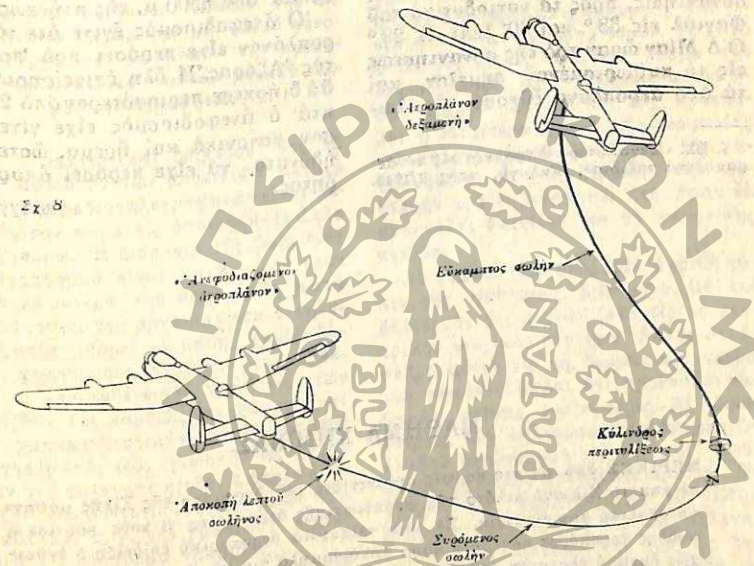
Σχ. 8. Τὸ ἀεροπλάνον - δεξαμενὴ στρέφεται διὰ νὰ ἐπιστρέψῃ εἰς τὴν βάσην του καὶ ἀποχωρίζεται ἀπὸ τοῦ ἀνεφοδιασθέντος πλέον ἀεροπλάνου διὰ τῆς ἀποκοπῆς τοῦ λεπτοῦ σωλήνος τοῦ ἀνεφοδιαζομένου ἀεροπλάνου.
