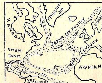
Χάρτης του Βορείου Ατλαντικού όπου διακρίνεται ή κίνηση του Ρεύματος μεταξύ Αμερικής - Ευρώπης - Αφρικής.
