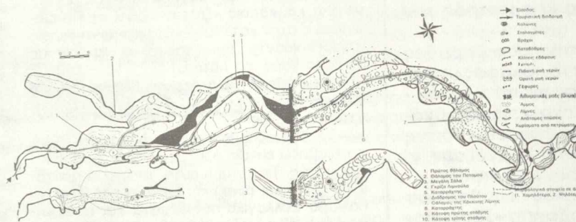
Σχέδιο του σπηλαίου Ανεμότρυπα Πραμάντων Ιωαννίνων. Μετρήσεις - Αποτύπωση: Α. Πετροχειλίου.
