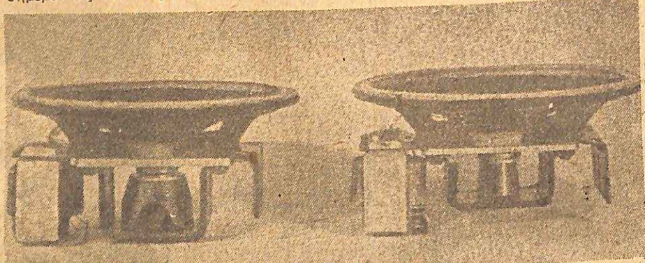
Τὰ νέα μαγνητικά κράματα : Δύο μεγάλων τῆς αὐτῆς ἰσχύος. Ἀριστερά, με συνήθη μαγνήτην. Δεξιά με μαγνήτην ἀπὸ τὸ νεὸν κράμα
