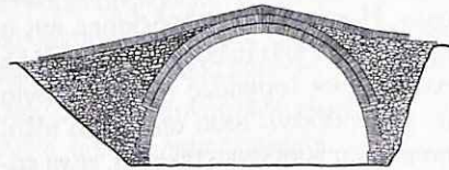
(Φωτ. 27-6) Η «γέφυρα Πεκλαρίου Καραγιάννη» σε αποτύπωση και σχέδιο του 1988. Όψη κατόντης. Φαίνεται το ελλιπές βοηθητικό στεφάνι του τόξου. [Πηγή: "Τα πετρογιόφυρα της Ηπείρου", Ιωάννινα 2012/3, της ΥΝΜΤΕΗ (Περιφέρεια Ηπείρου), σελ. 78].
