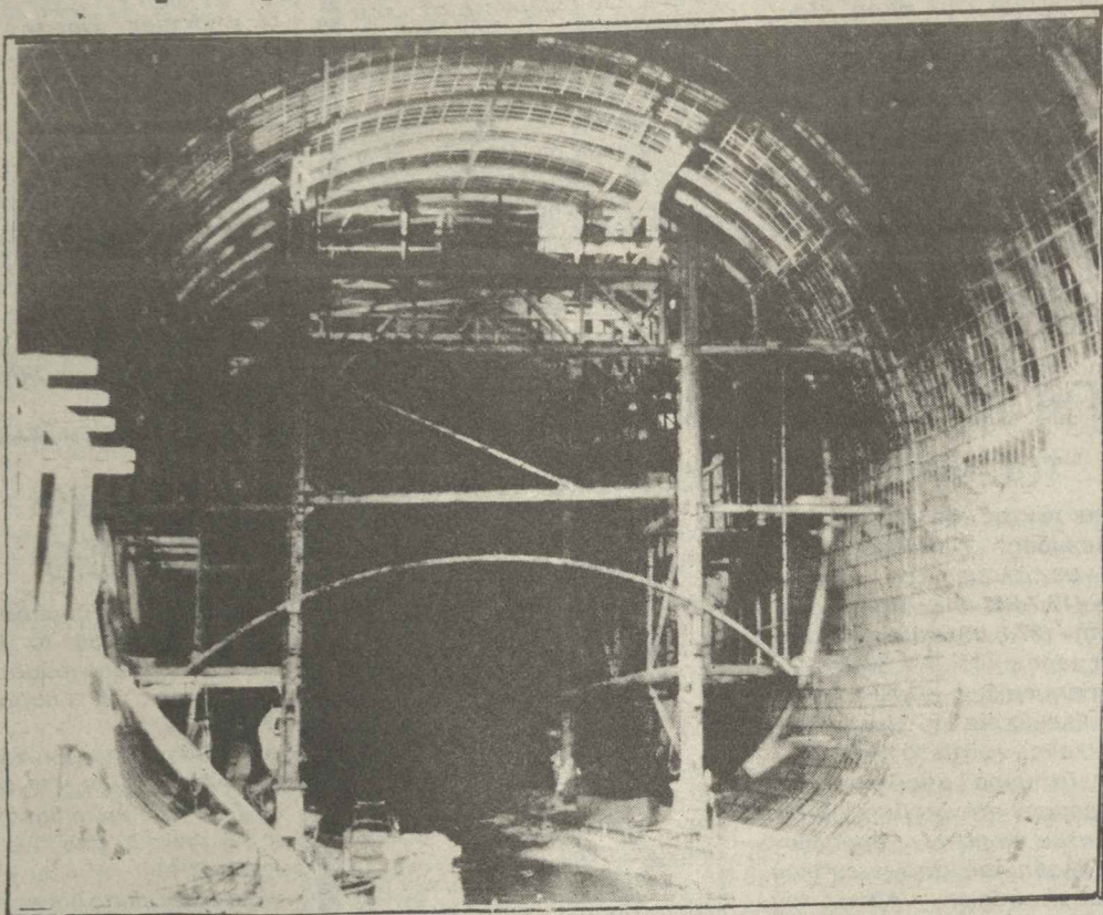
Μιά άποψη από τη σήραγγα εκτροπής του Αχελώου στη Συκιά
