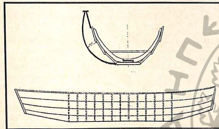
Τρόπος δημιουργίας πλωτήρων με την τοποθέτηση πρόσθετων νομείων και πετωμάτων στη "Σκνίπα"
