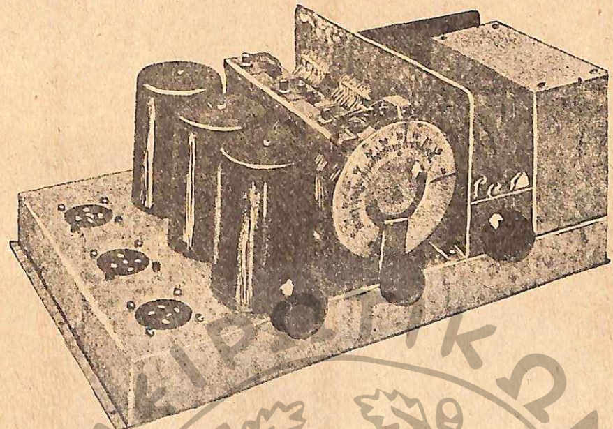
Ἡ γενικὴ ὅψις μετὰ τὴν συναρμολόγησιν τοῦ εἰς τὸ προηγούμενον τεύχος δημοσιευθέντος δέκτου.
