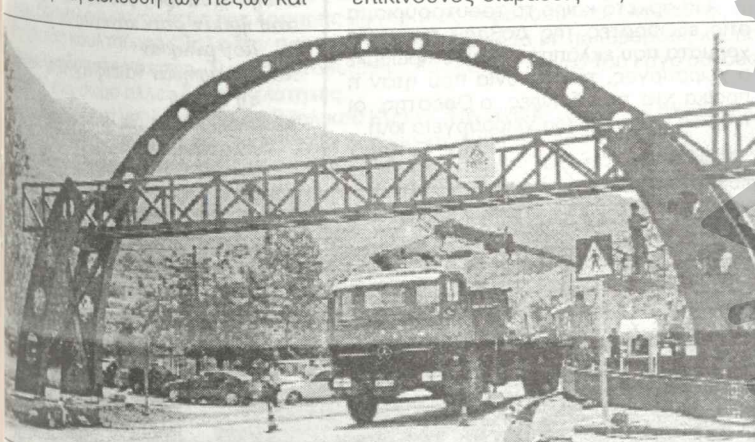
Πεζογέφυρα που κατασκευάστηκε κοντά στη Μεταμόρφωση. Παρόμοιες γέφυρες για ασφαλή διέλευση των πεζών θα γίνουν και σε άλλα σημεία του εθνικού οδικού δικτύου.
