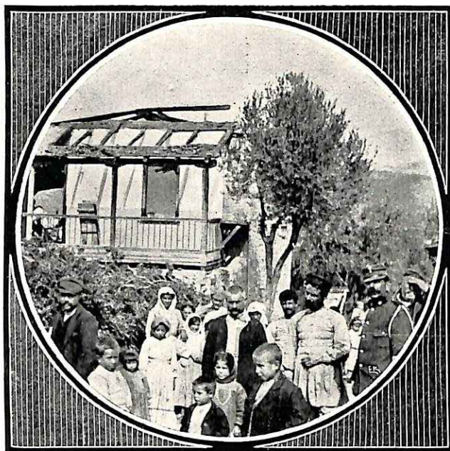
ΟΙ ΣΕΙΣΜΟΙ ΤΩΝ ΘΗΒΩΝ
