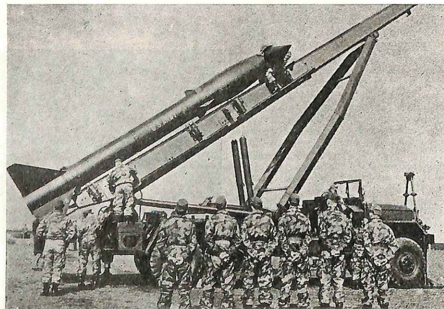
Τὸ πρῶτον γερμανικὸν τάγμα διὰ τὸν χειρισμὸν πυραύλων μέσον βεληγκοῦς «Τίμιος Τζὼν» ἤρχισεν ἀσκήσεις ἐκτοξεύσεως βλημάτων εἰς Ἑσβιάλερ τῆς Δ. Γερμανίας
