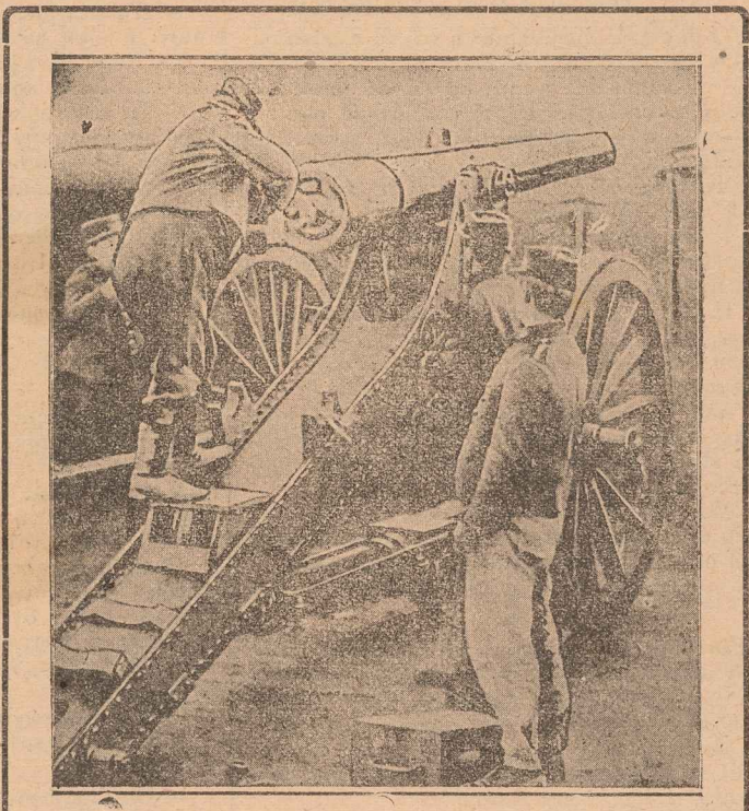
Μέγα τηλεβόλον, εκ τών τελειοποιηθέντων εσχάτως και χρησιμοποιούμενων κατά τὸν Ενωπαϊκόν πόλεμον. Παρίσταται την στιγμήν της σκοπεύσεως επί του πεδίου μιάς τών προσάτων μαχών.
