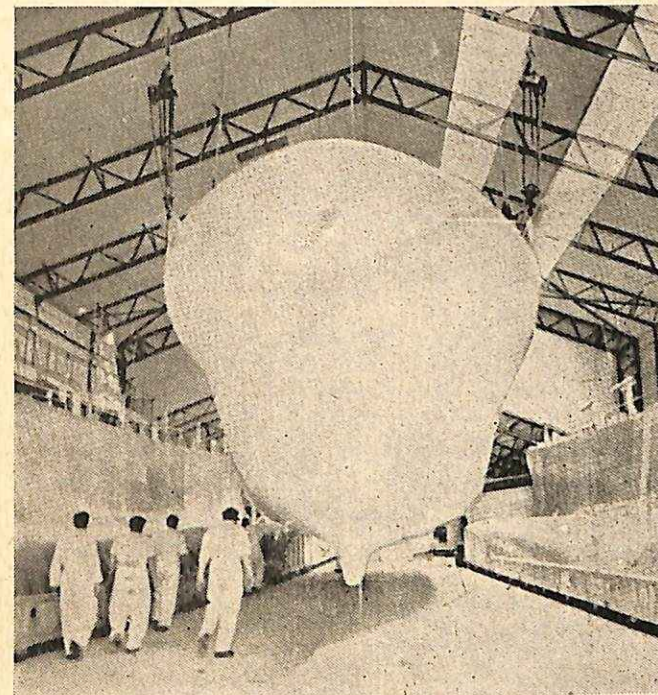
Τελευταίως κατεσκευάσθη εἰς τὰ ναυπηγεῖα τοῦ Πόρτσμουθ τὸ πρῶτον σκάφος ἀπὸ πλαστικὸν γυαλὶ διὰ λογαριασμὸν ἀμερικανικῆς ἐταιρίας. Εἰς τὴν φωτογραφίαν τὸ σκάφος μήκους 67 ποδῶν εἰς τὰ ναυπηγεῖα τοῦ Πόρτσμουθ ἀποπερατοῦται ταχύτατα διὰ νὰ ἀποσταλῇ τὸ συντομώτερον εἰς Ἡν. Πολιτείαν.
