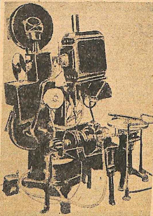
Μηχάνημα τύπου «Βιταφόν - Μούβιτον» διὰ τὴν προβολὴν συγχρόνως ἡχου καὶ εἰκόνων.
