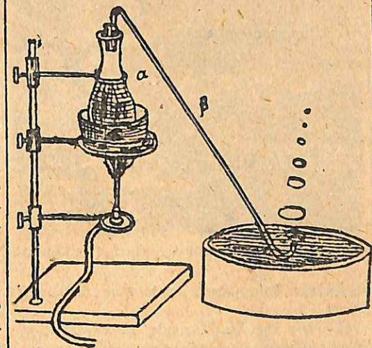
Συσκευή πρὸς παραγωγὴν φωσφίνης.
